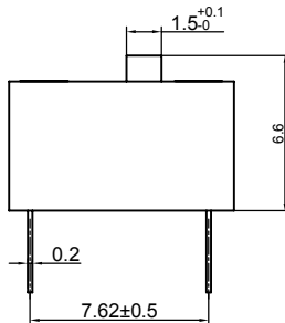
高推钮 (E)
